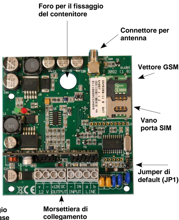
Fig. 2 - immagine scheda elettronica T 3092
